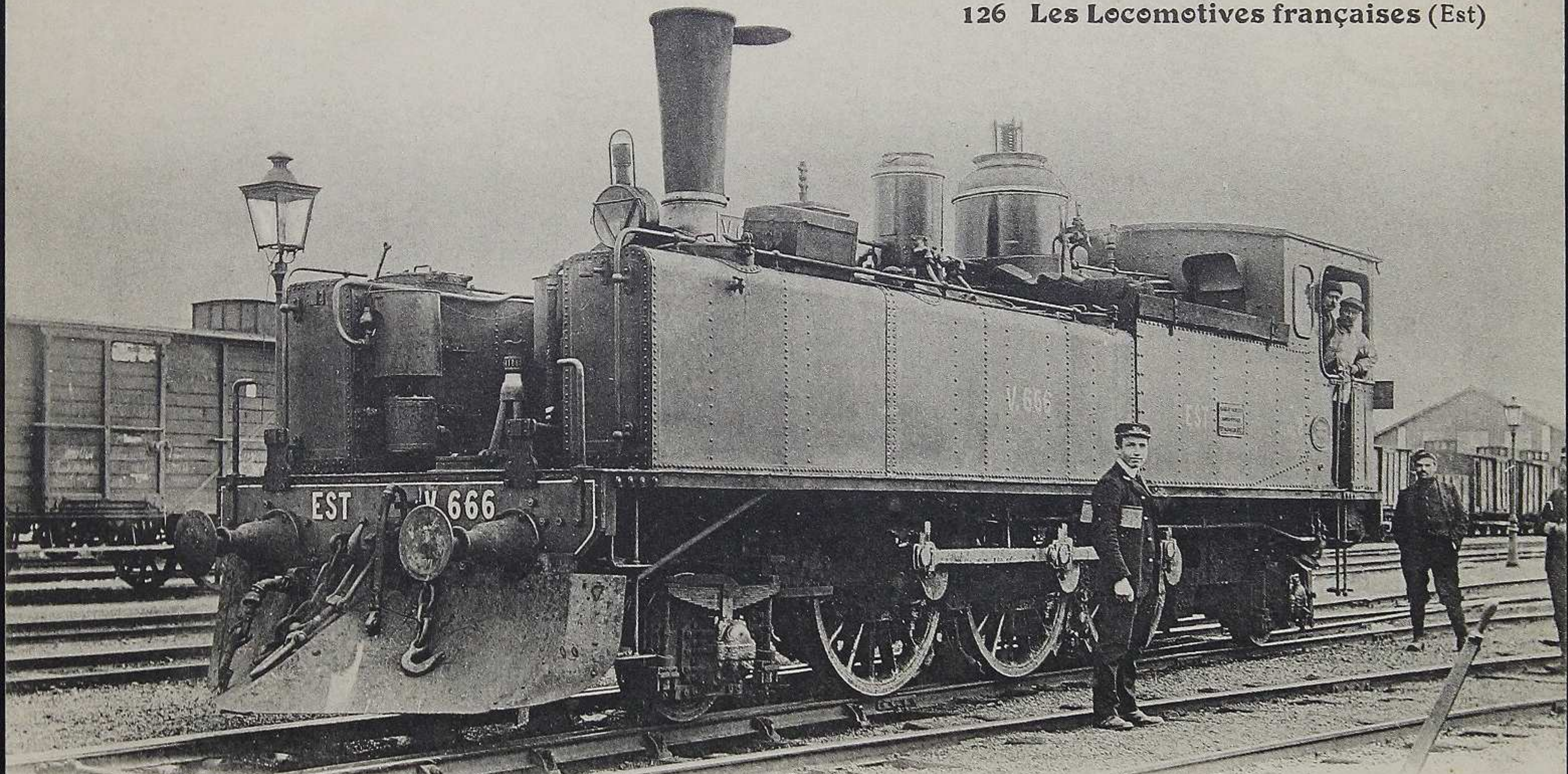
Machine-tender N° V. 666, à vapeur saturée, simple expansion, tiroirs plans, mécanisme intérieur, 3 essieux accouplés compris entre 2 bissels, pour trains de banlieue (Série V. 613 à 683, construite en 1881, transformée en 1905-1911). Cette machine est munie d'un chasse-neige amovible
