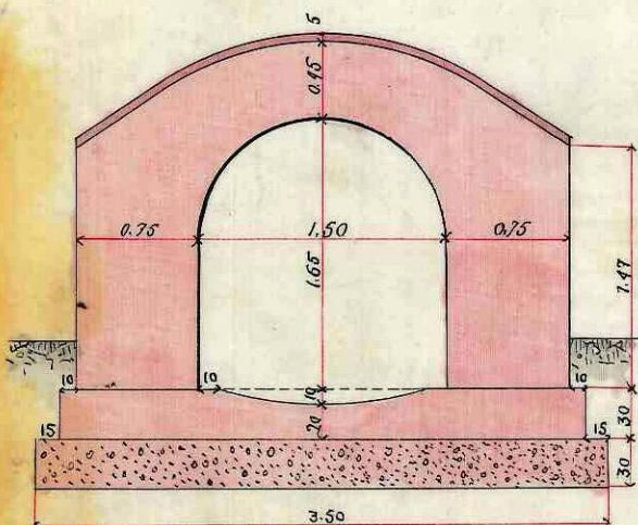
Coupe transversale dans la long. de 5 m 00 à partir des têtes
