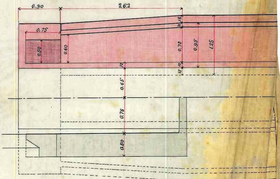
Plans des fondations
