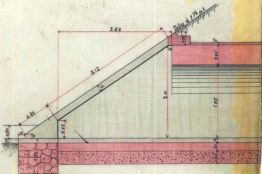
Coupes Longitudinales
